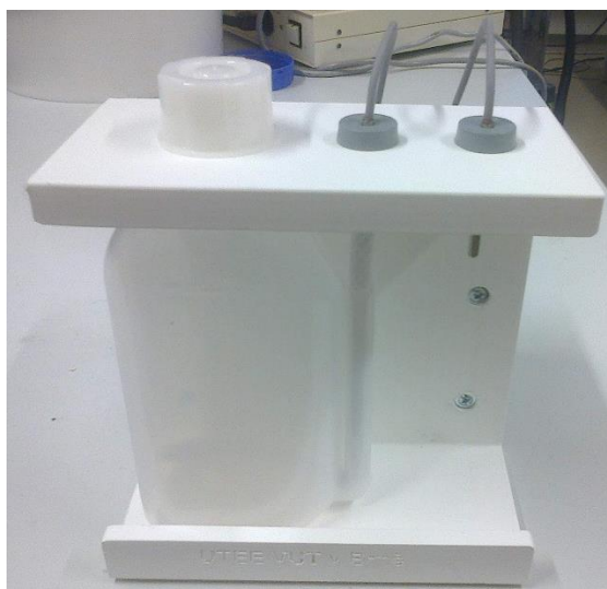
Obr. 1: Funkční vzorek psychrometru.
